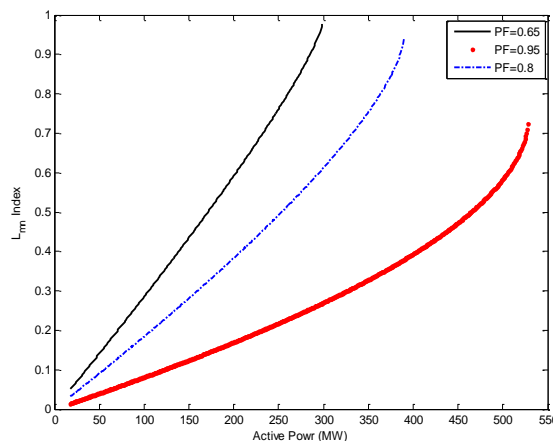
شکل ۸. تغییرات شاخص L_{mn} به ازای بارگذاری‌ها و ضرایب توان
