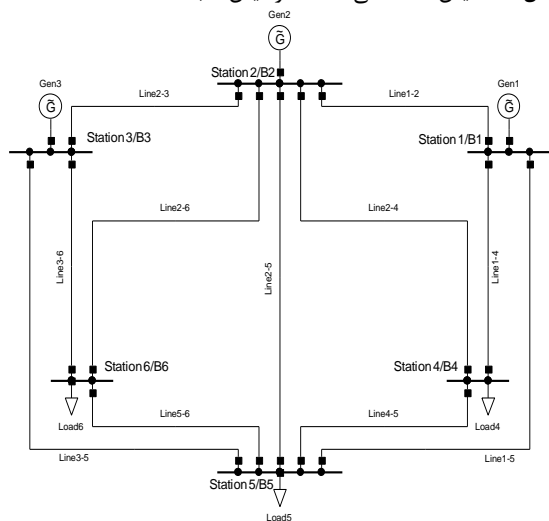
شکل ۷. نمایش تک خطی سامانه آزمایش ۶ باسه
