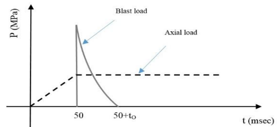
شکل ۷. مراحل اعمال بار محوری و بار انفجار بر ستون در نرم‌افزار LS-DYNA
